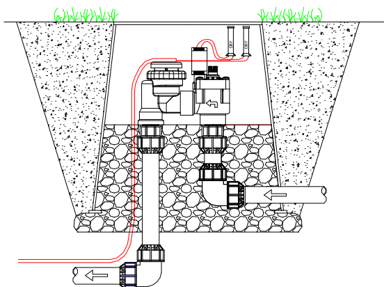
Schéma uložení ASV – 075 – 3/4" v šachtici
