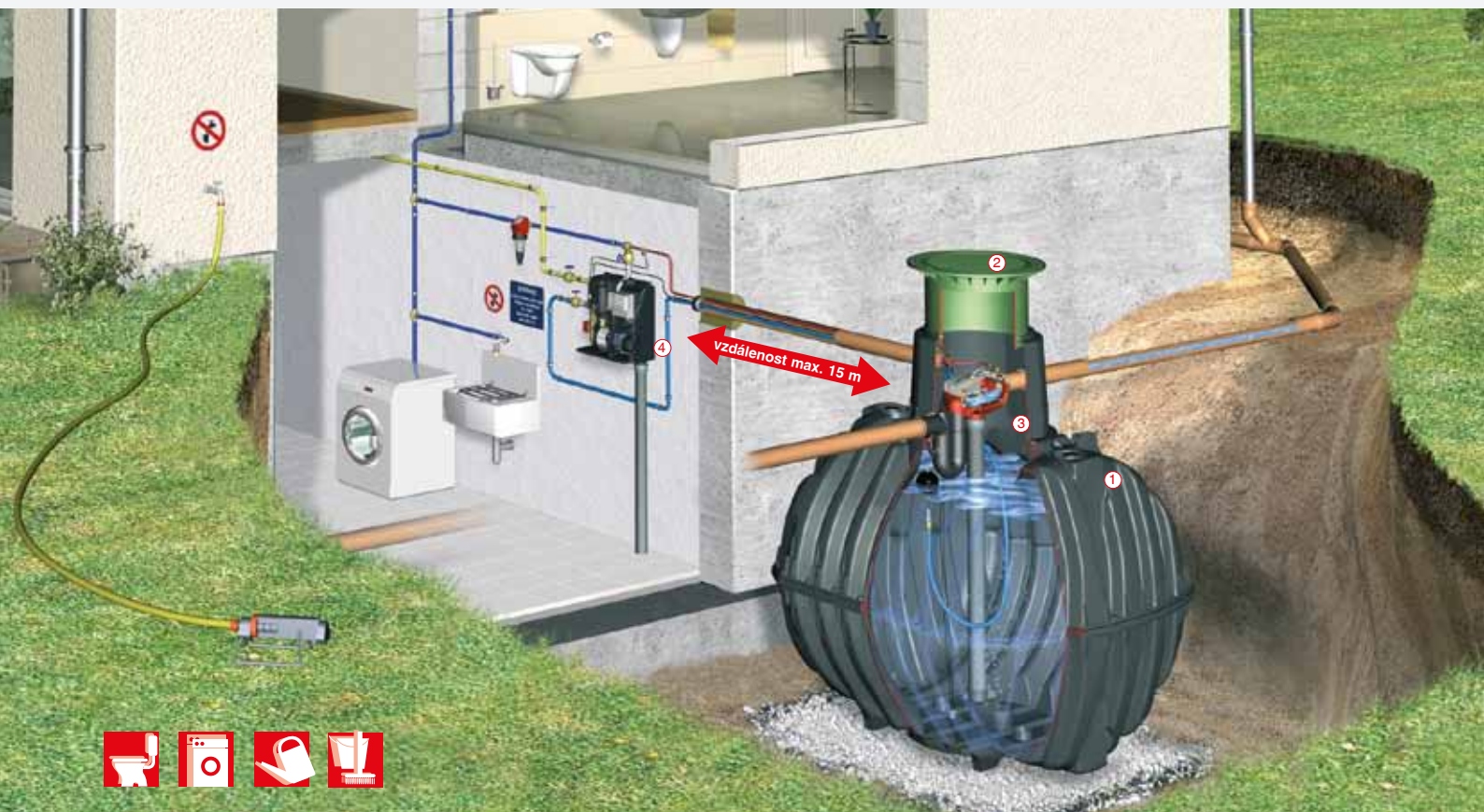
Sestava podzemní nádrže Carat Professionell s pochozím poklopem nádrže
